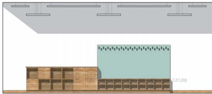
elevation A
